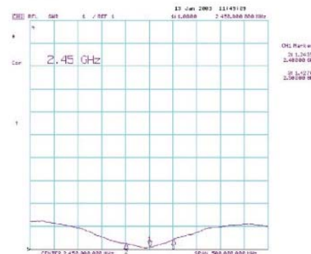
VSWR
